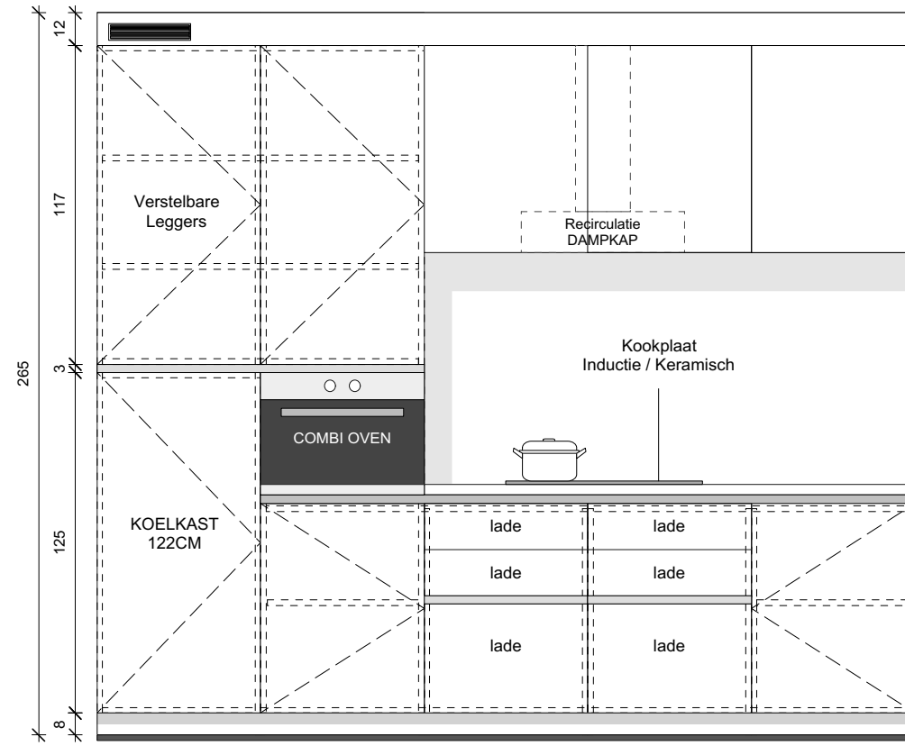
AANZICHT - KEUKEN
