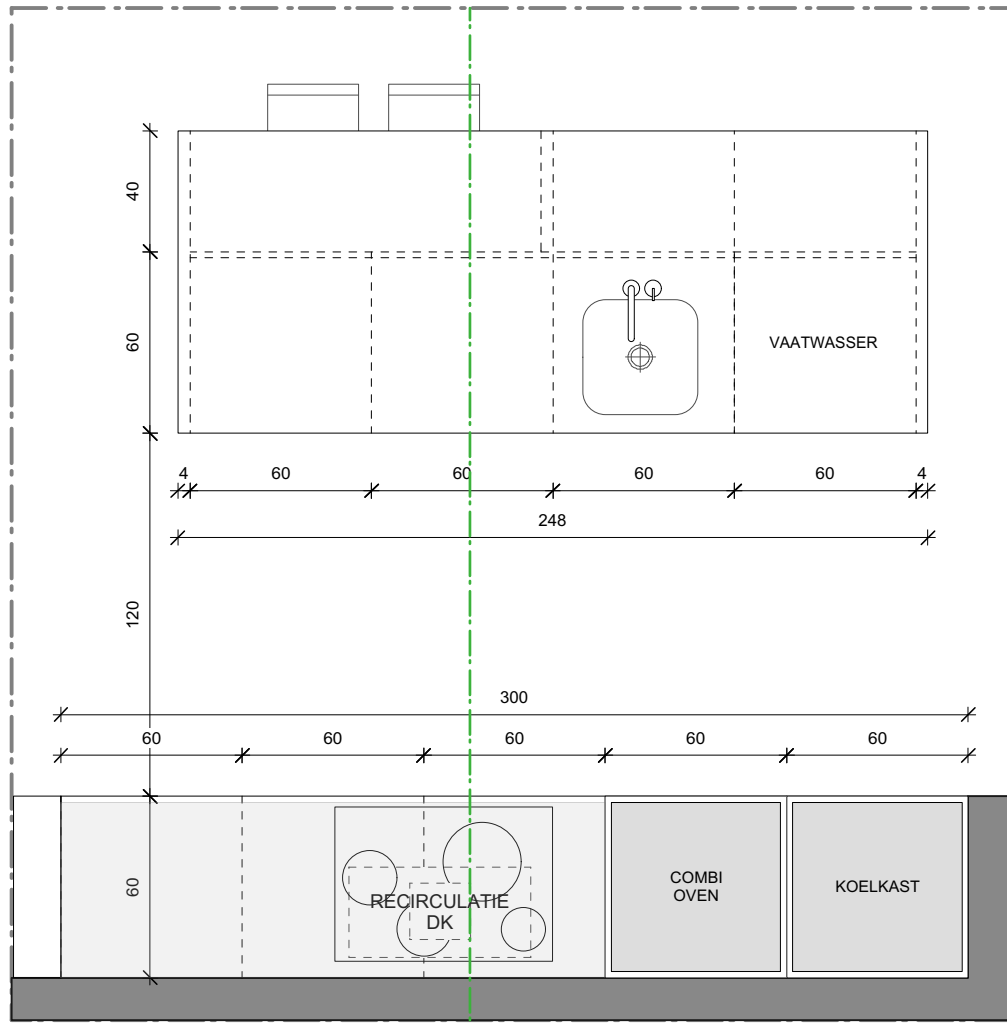
GRONDPLAN KEUKEN
