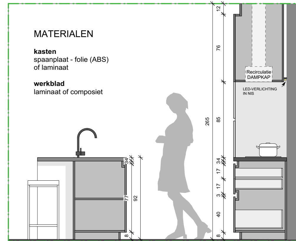
SNEDE KEUKEN
