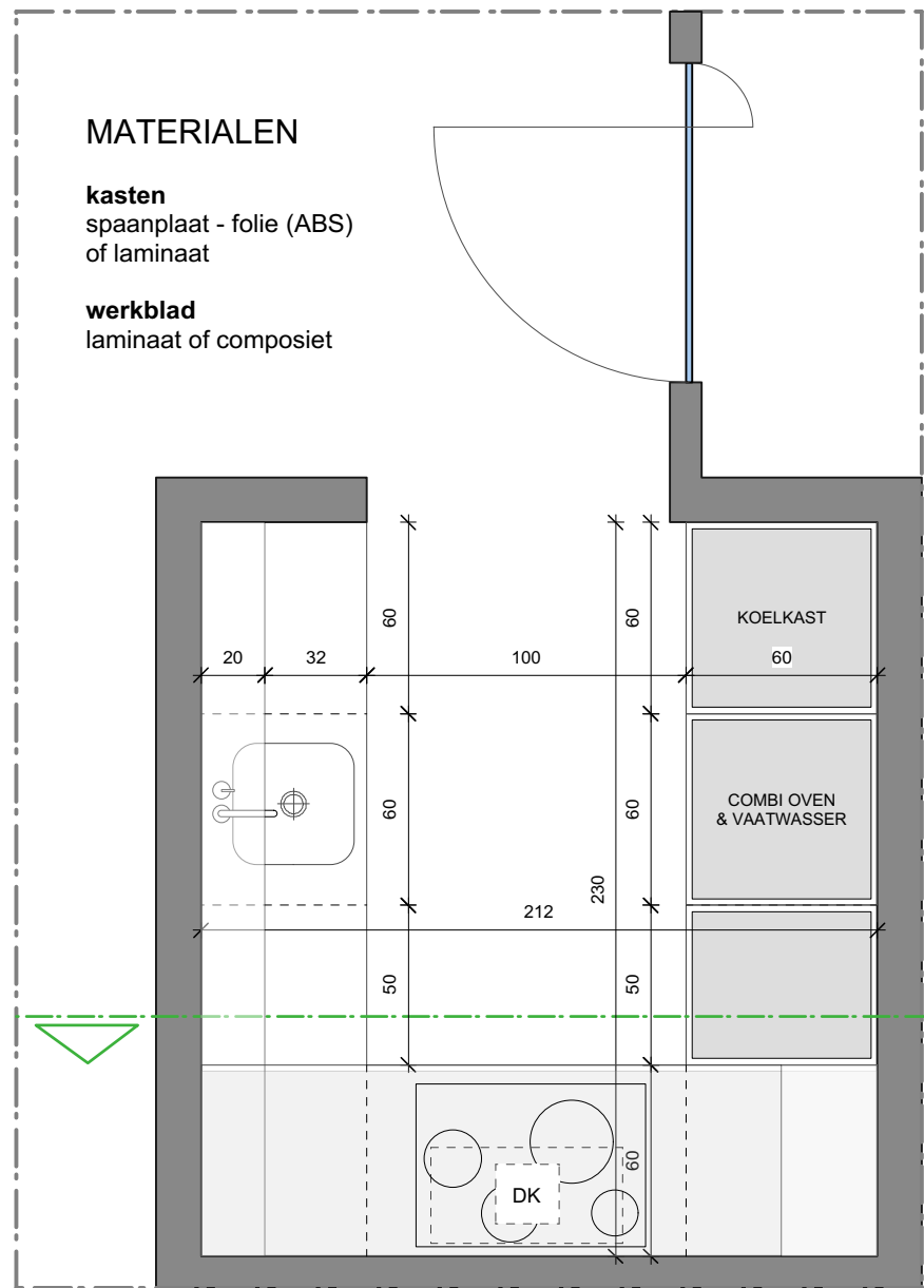
GRONDPLAN KEUKEN
