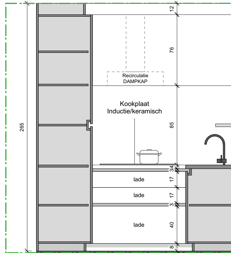
SNEDE - KEUKEN
