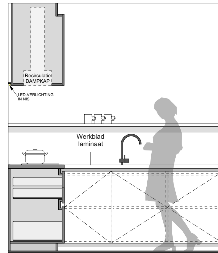
AANZICHT & SNEDE - KEUKEN
