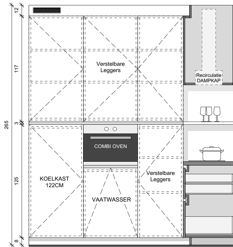
AANZICHT & SNEDE - KEUKEN
