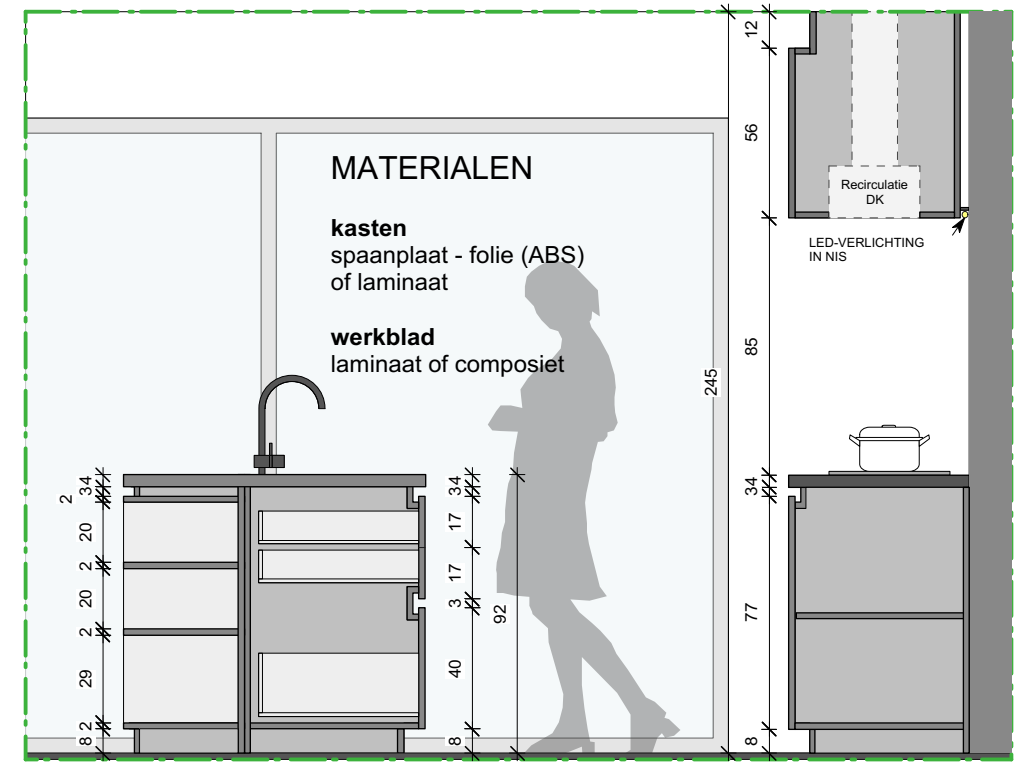
SNEDE KEUKEN
