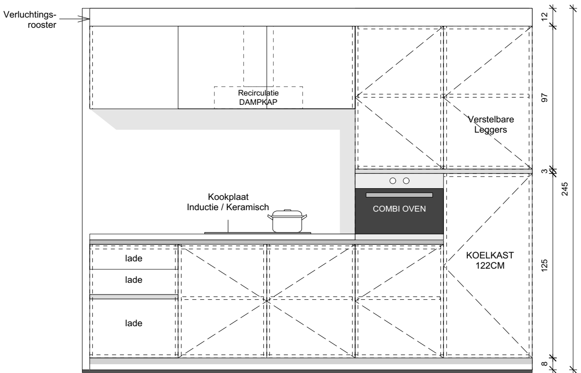
AANZICHT - KEUKEN
