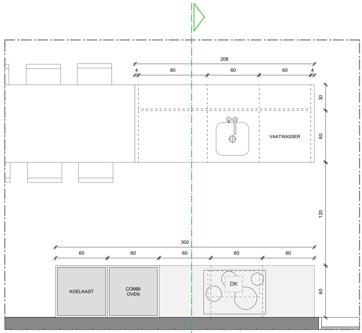
GRONDPLAN KEUKEN
