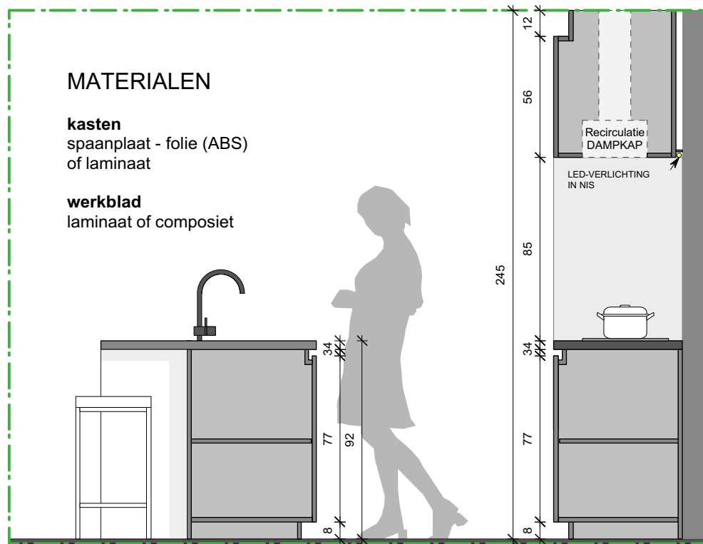
SNEDE KEUKEN
