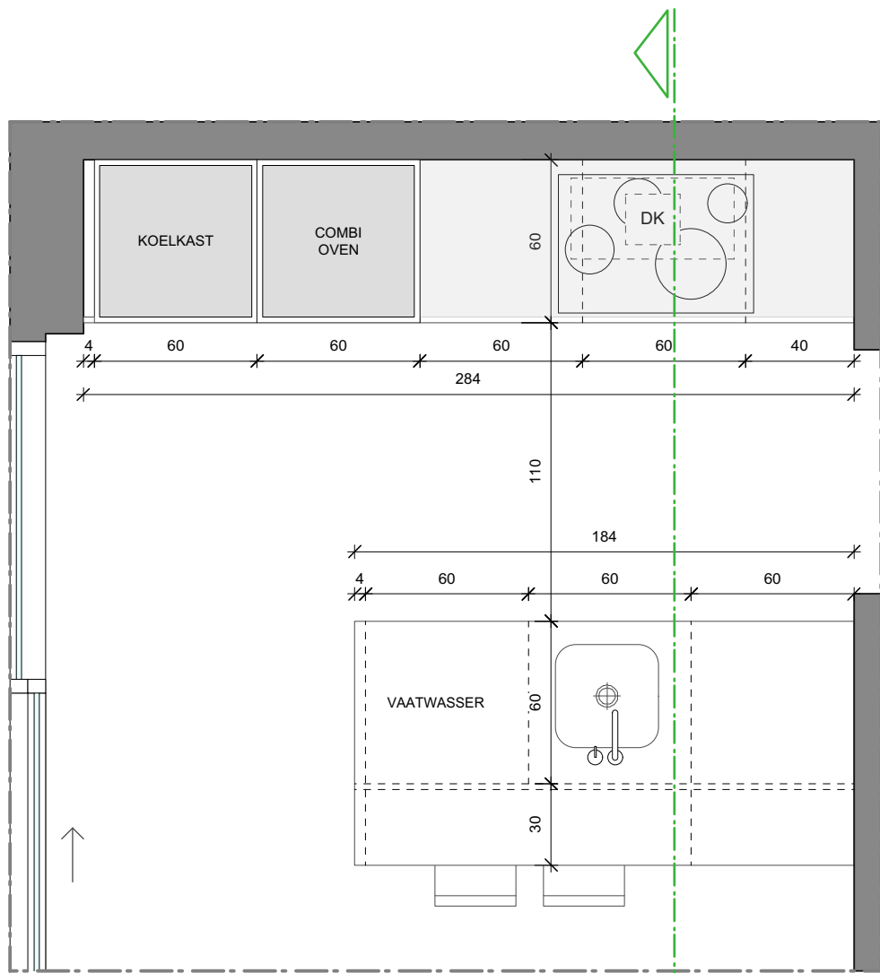
GRONDPLAN KEUKEN
