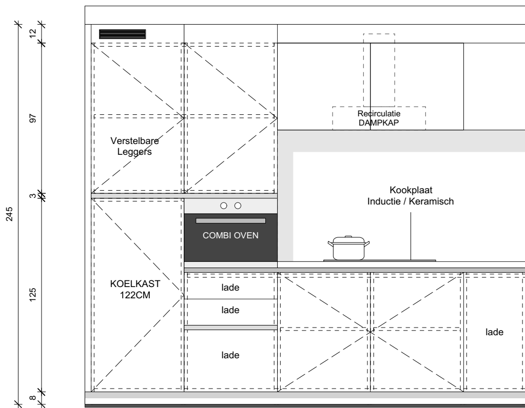
AANZICHT - KEUKEN
