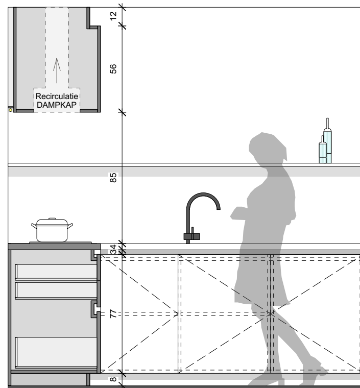
AANZICHT & SNEDE - KEUKEN
