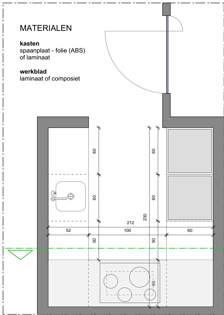
GRONDPLAN KEUKEN
