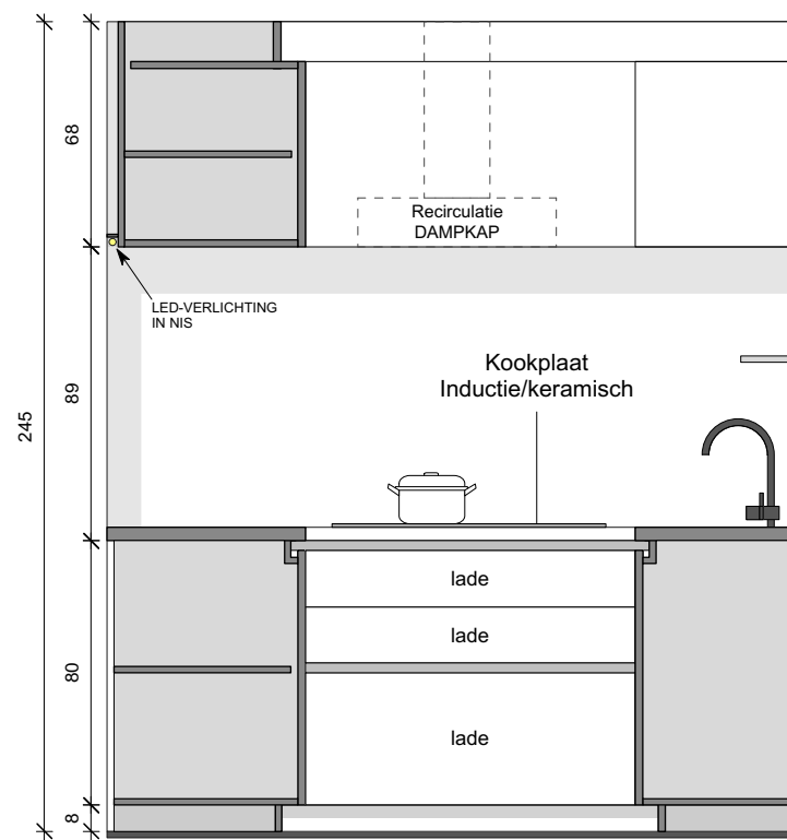
SNEDE - KEUKEN
