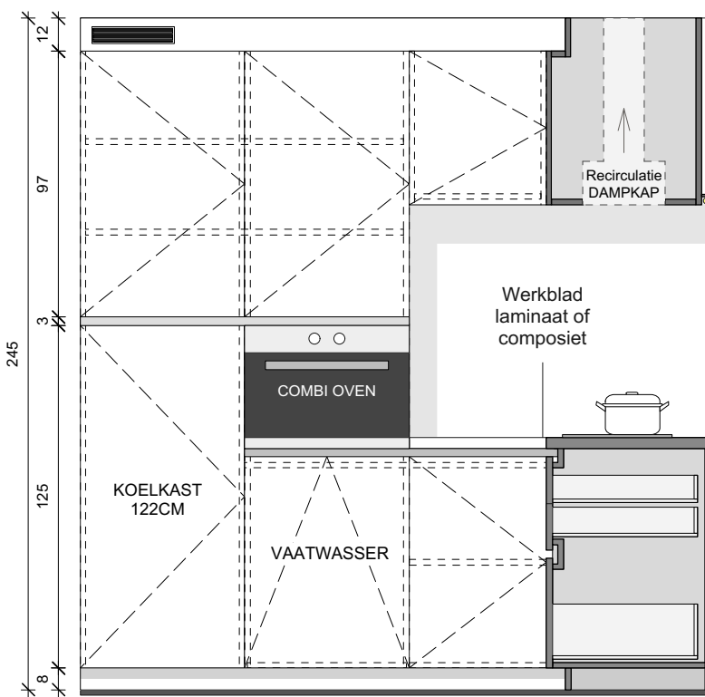
AANZICHT & SNEDE - KEUKEN
